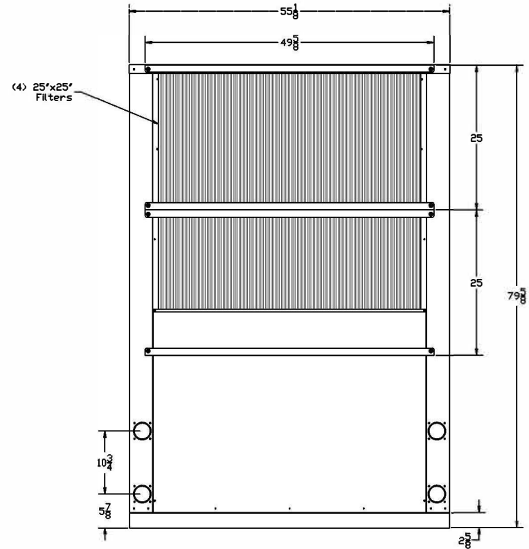
Elevation "C"
