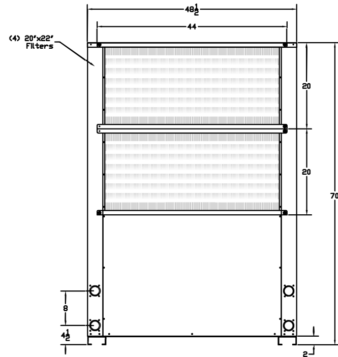
Elevation 'C'
