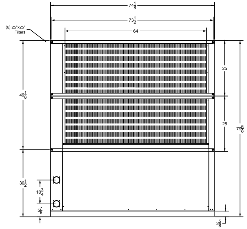
Elevation "C"
